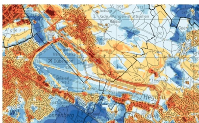
GIS-ZH: Wärmeinselleffekt (Screenshot 4.8.2022)
